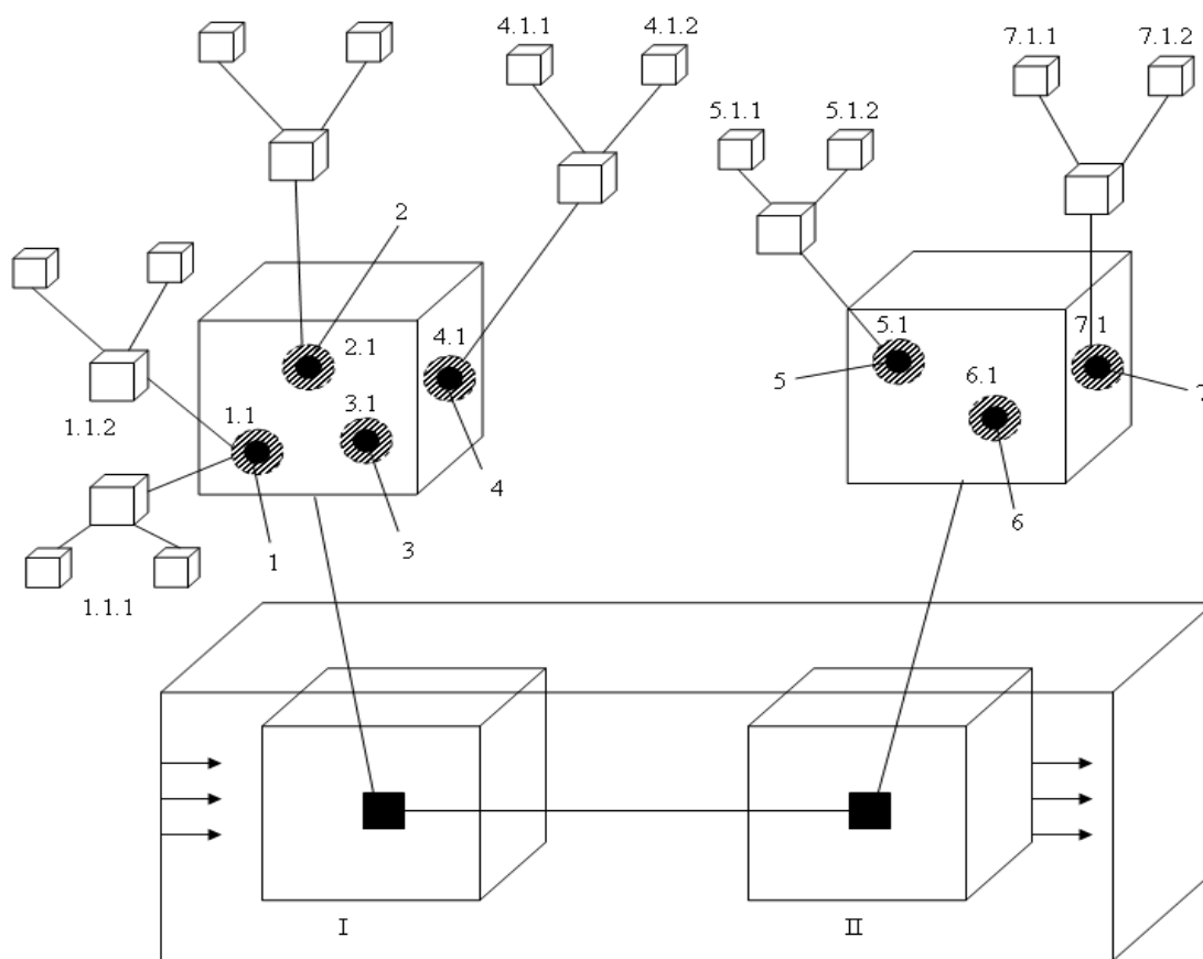
Рис. 5.1. Декодовані "чорні скрині":
