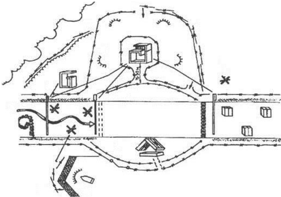
Мал. 1. Типовий план блокпоста
