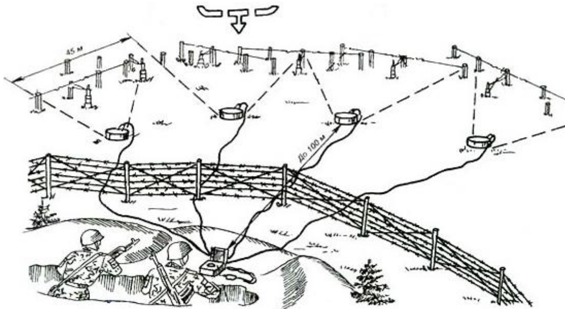
Мал. 2. Зразок облаштування керованого мінно-вибухового загородження
