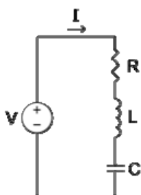
Рис.2. Еквівалент послідовного R,L,C коливального контуру частотного міношукача, де: V – напруга в контурі, I – сила струму в контурі, R – внутрішній опір провідника, L – котушка індуктивності, C – конденсатор
