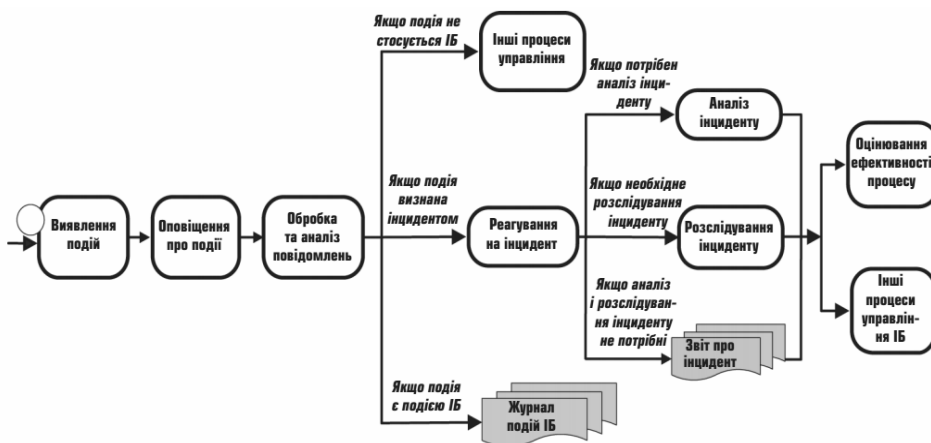
Рис. 3. Процес управління інцидентами інформаційної безпеки
