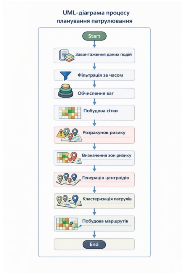
Рис. 2.7. Блок-схема алгоритму планування патрулювання
